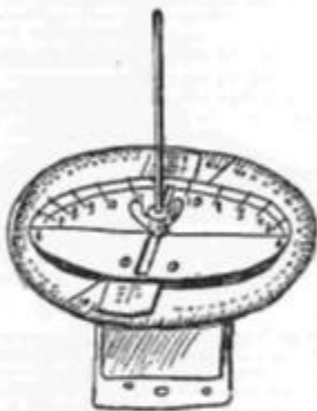
Schéma du compas solaire employé par le commandant Armand pour la traversée du Ténére
